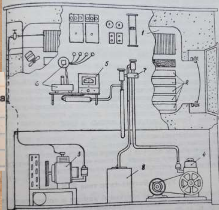
Схема однокамерного вакуумсушильного аппарата ( I вариант )
